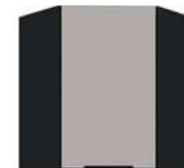
60x60 GN-72 1F (45°) S: 60x60 / W: 71,5 / G: 31 cm 2 paczki • waga: 27 kg
