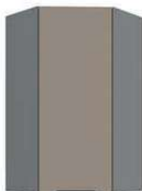
60x60 GN-108 1F (45°) S: 60x60 / W: 107,5 / G: 31 cm 2 paczki • waga: 36,5 kg
